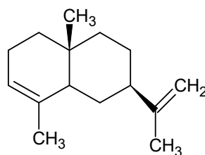
\alpha -selinene
